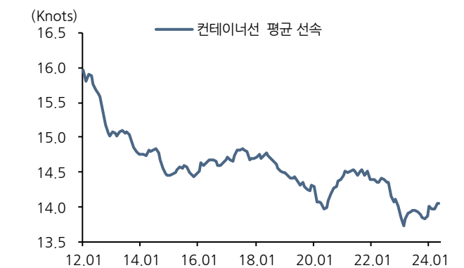
그림 70. 컨테이너선 평균 선속 추이
